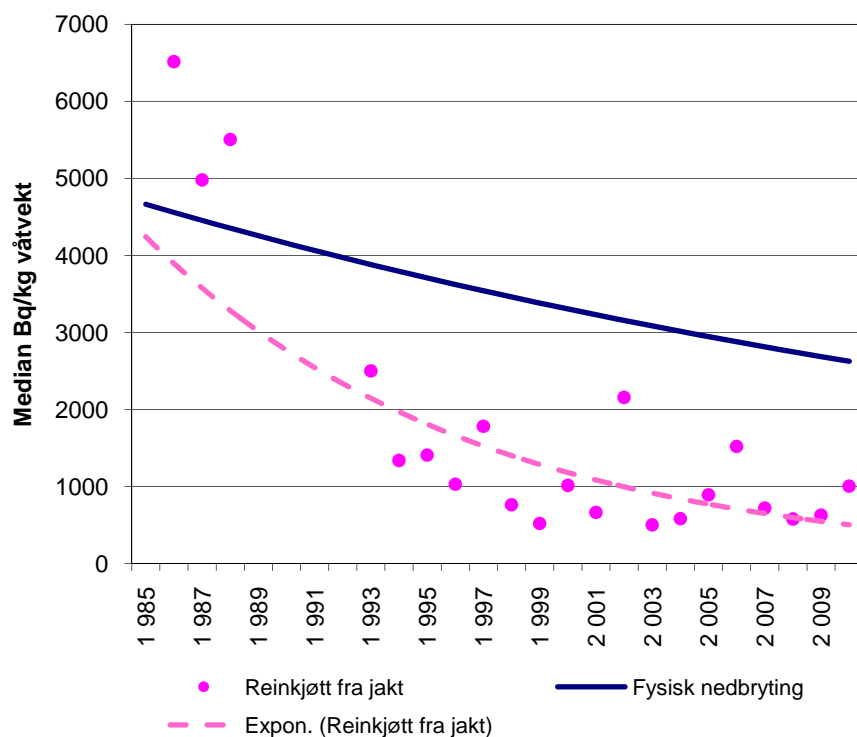
Figur 3.3. Endringen av Cs-137-aktiviteten i reinkjøtt i Nord-Rondane er vist for perioden 1986-2010. Verdiene er medianen av 5 til 18 årlige prøver. Den blå kurven øverst viser hva en kunne vente om fysisk omdanning av Cs-137 var den eneste årsak til nedgangen (fysisk halveringstid for Cs-137 er 30,1 år). En eksponentiell linje er tilpasset de observerte konsentrasjonene og indikerer en effektiv halveringstid i reinkjøtt på ca. 8,5 år for hele perioden.
