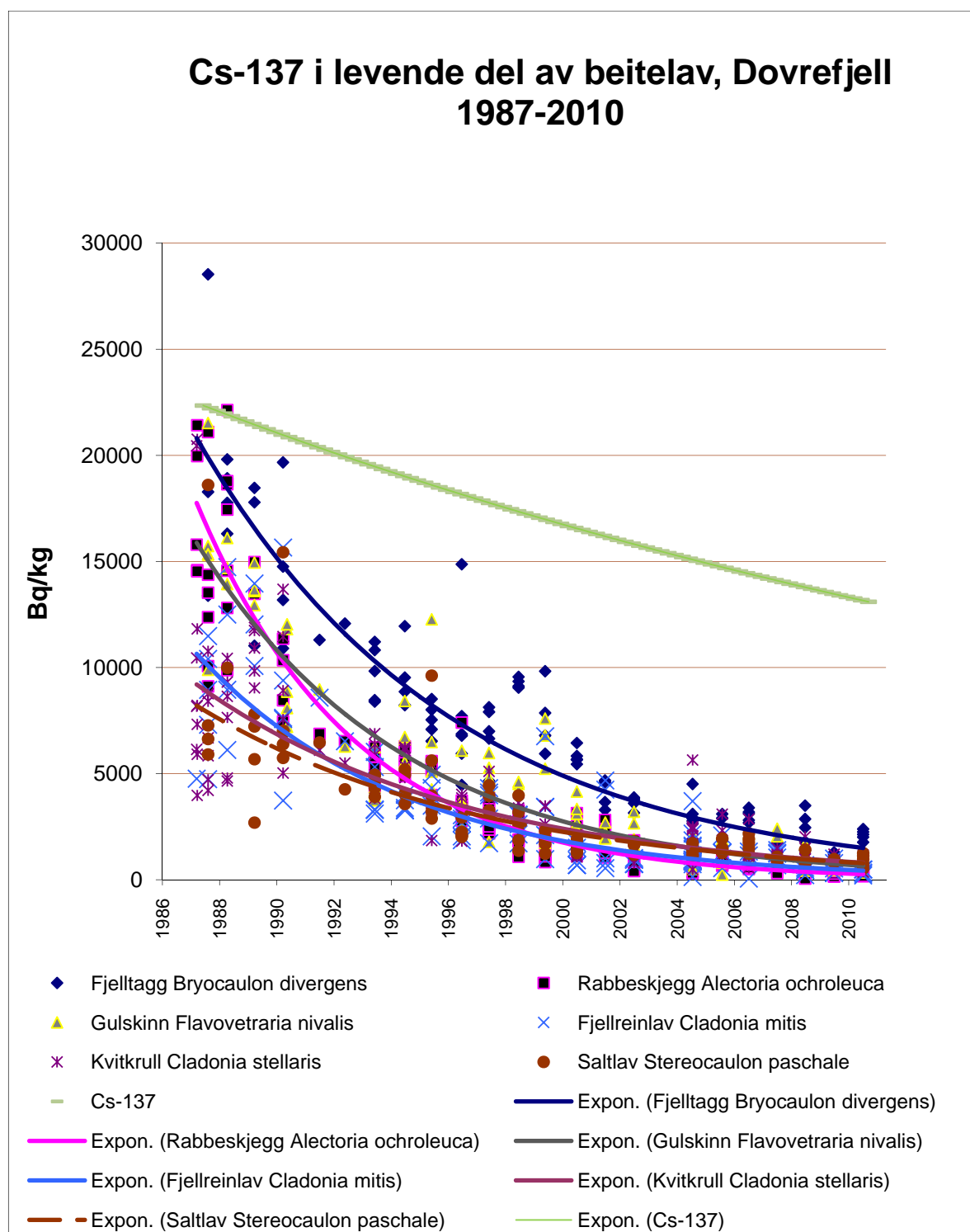
Figur 3.4. Endringen av Cs-137-aktiviteten i lavarter samlet på et prøvetakingsfeltet Grønbakken (GRB) 4 km sør for Kongsvold fjeldstue i perioden 1987-2010. Rekkefølgen reflekterer artenes økende krav til beskyttelse mot vindslitasje og tørke. Den øverste grønne kurven viser forløpet av fysisk nedbryting av Cs-137. Denne nukliden har en halveringstid på 30,1 år.
