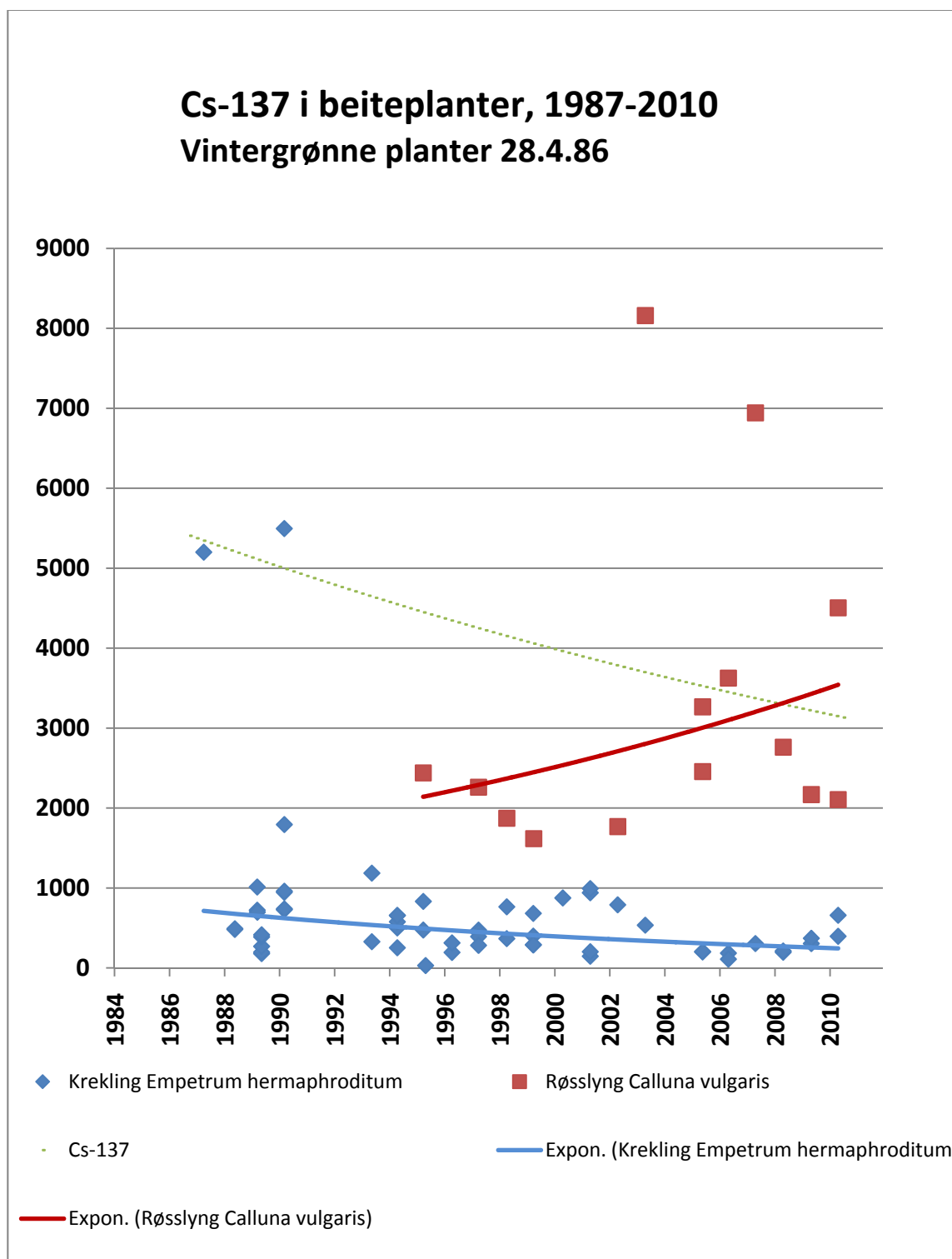
Figur 3.6. Endringen av Cs-137-aktiviteten i beitevekster samlet på et prøvetakingsfelt nær Bergedalsbekken Nord-Rondane (ST1) i perioden 1987-2010. Artene vokser med svak snøbeskyttelse, på vindrabb. Begge arter er vintergrønne med grunt rotsystem. Den prikkede kurven viser forløpet av fysisk nedbryting av Cs-137. Denne nukliden har en halveringstid på 30,1 år.
